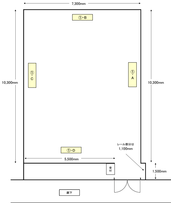
ギャラリー① 平面図
