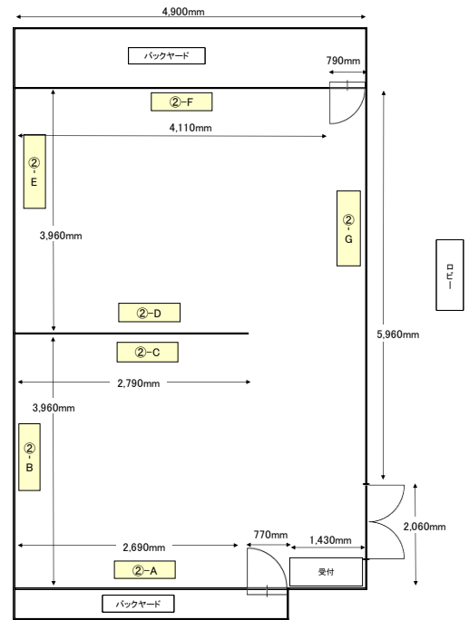
ギャラリー② 平面図
